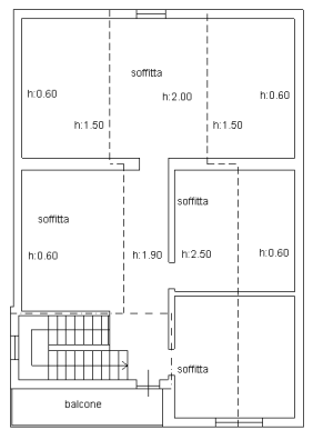
PIANO PRIMO
